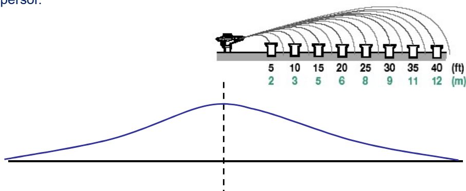
Diagrama pluviométrico típico de um aspersor funcionando correctamente
