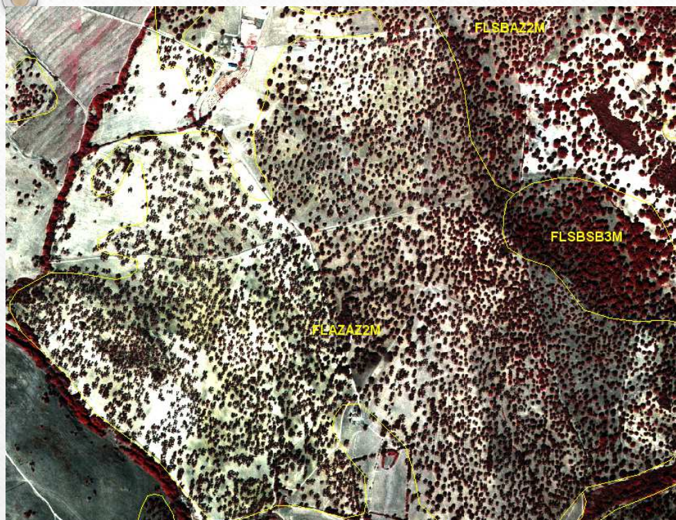
Figura 3. Delimitação de manchas de sobreiro e de azinheira, com particular destaque para a distinção de povoamentos puros e mistos de ambas as espécies..
