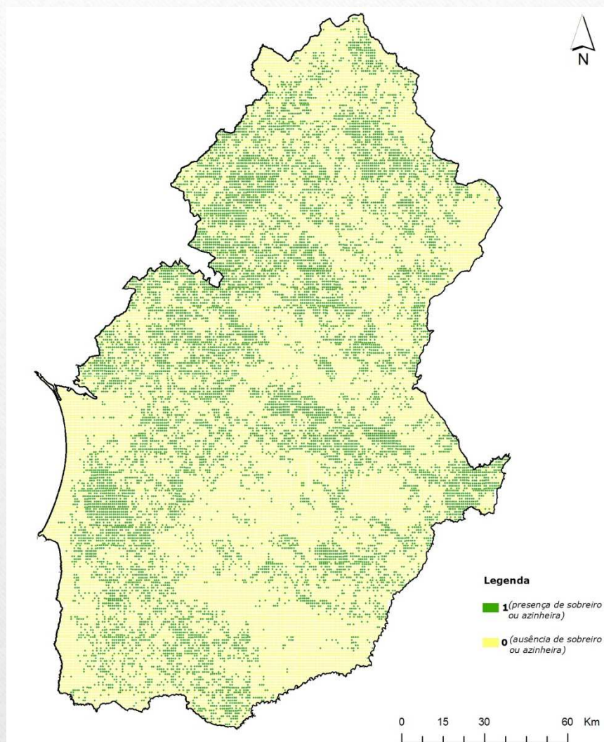
Figura 1. Fotopontos do Inventário Florestal Nacional codificados sob a forma de indicatriz.
