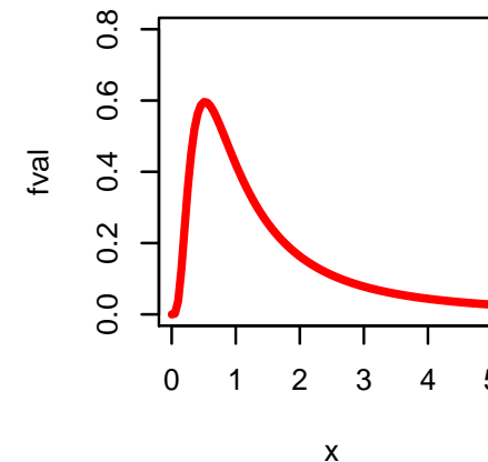
f. densidade da F_{(15,3)}
