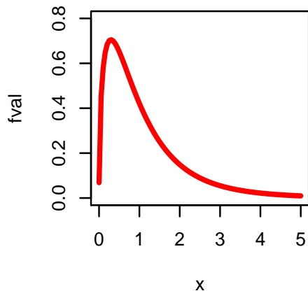
f. densidade da F_{(3,15)}
