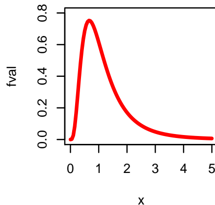
f. densidade da F_{(10,10)}
