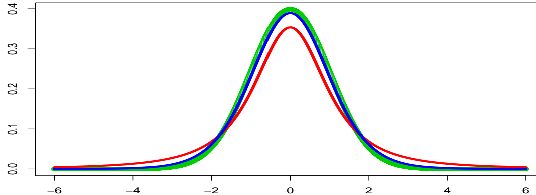
Gráficos da função densidade de uma v.a. com distribuição N(0, 1) , t_{(2)} e t_{(10)} .
