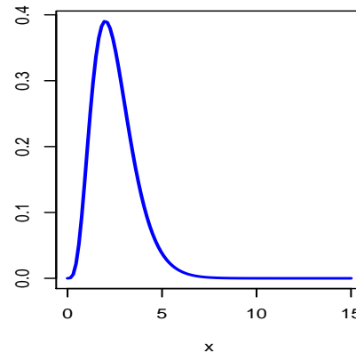
f. densidade da Qui-quadrado(n=10)
