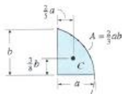
Área semiparabólica
