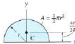
Área semicircular
