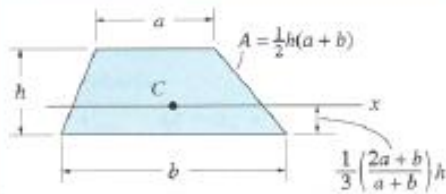
Área trapezoidal
