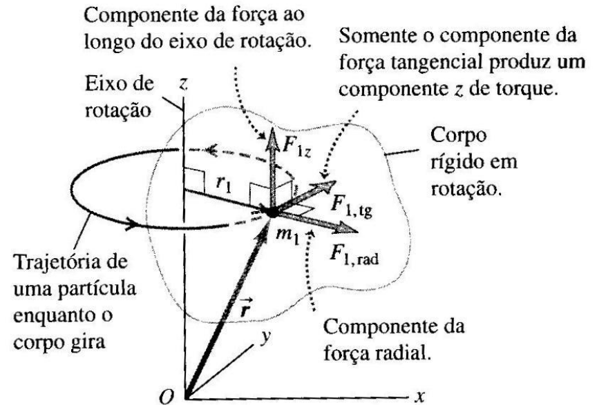
Figura 10.6 Enquanto um corpo rígido gira em torno do eixo z , uma força resultante \mathbf{F}_1 atua sobre uma partícula do corpo. Somente o componente da força F_{1,tg} pode afetar a rotação, porque somente ele exerce um torque em torno de O com um componente z (ao longo do eixo de rotação).
