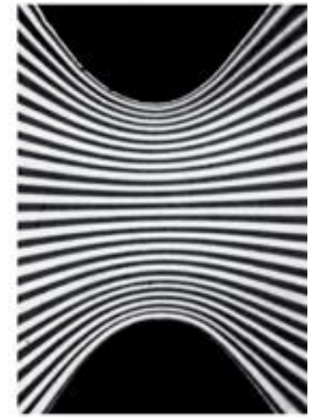
d) Escoamento numa secção de um canal com as paredes de forma irregular
