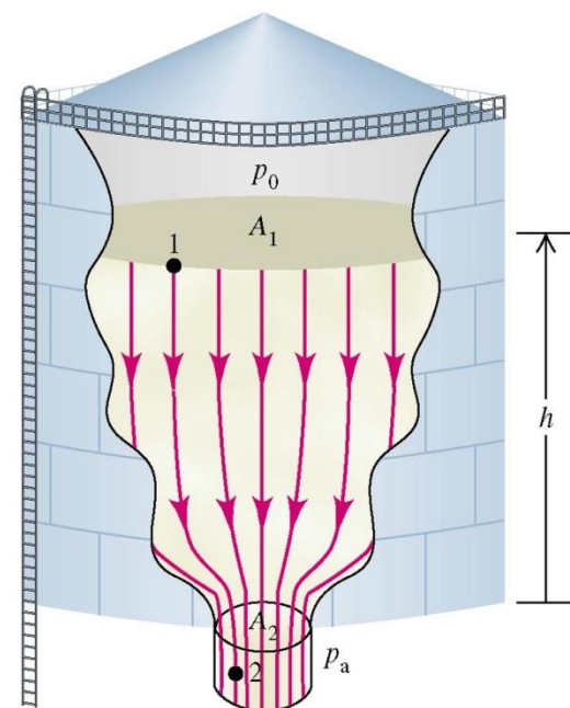
FIGURA 14.24 Esquema para calcular a velocidade de efluxo da gasolina que escoar pela parte inferior do tanque de armazenamento.
