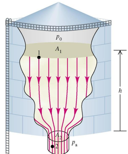
FIGURA 14.24 Esquema para calcular a velocidade de efluxo da gasolina que escoo pela parte inferior do tanque de armazenamento.
